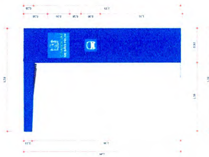
5 VISTA LATERAL DIREITA PONTO DE ÔNIBUS ESCALA 1:20
