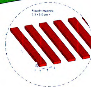
9 DETALHE RIPA DE MADEIRA ESCALA 1:5
