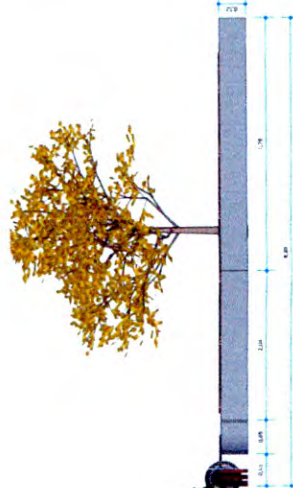
6 VISTA LATERAL ESQUERDA BANCO DE CONCRETO 05 ESCALA 1:50
