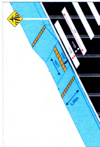
3 DETALHE RAMPA
